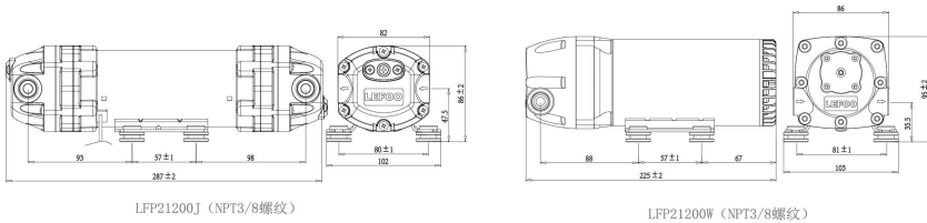
LFP21200W (NPT3/8螺纹)
