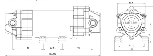
LFP21500W (NPT3/8螺纹)
